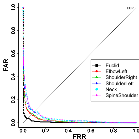
図 12 ROC カーブ
